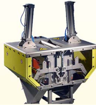
自清理磁板式管道除铁器
