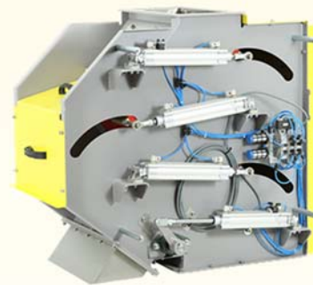
自清理驼峰式管道除铁器
